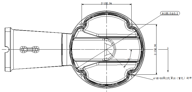
视图 A-A
