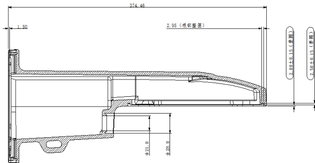
视图 A-A
